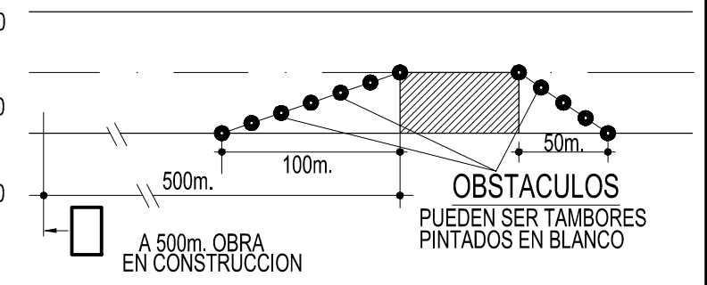
SEÑALIZACION DE OBRAS EN CONSTRUCCION
