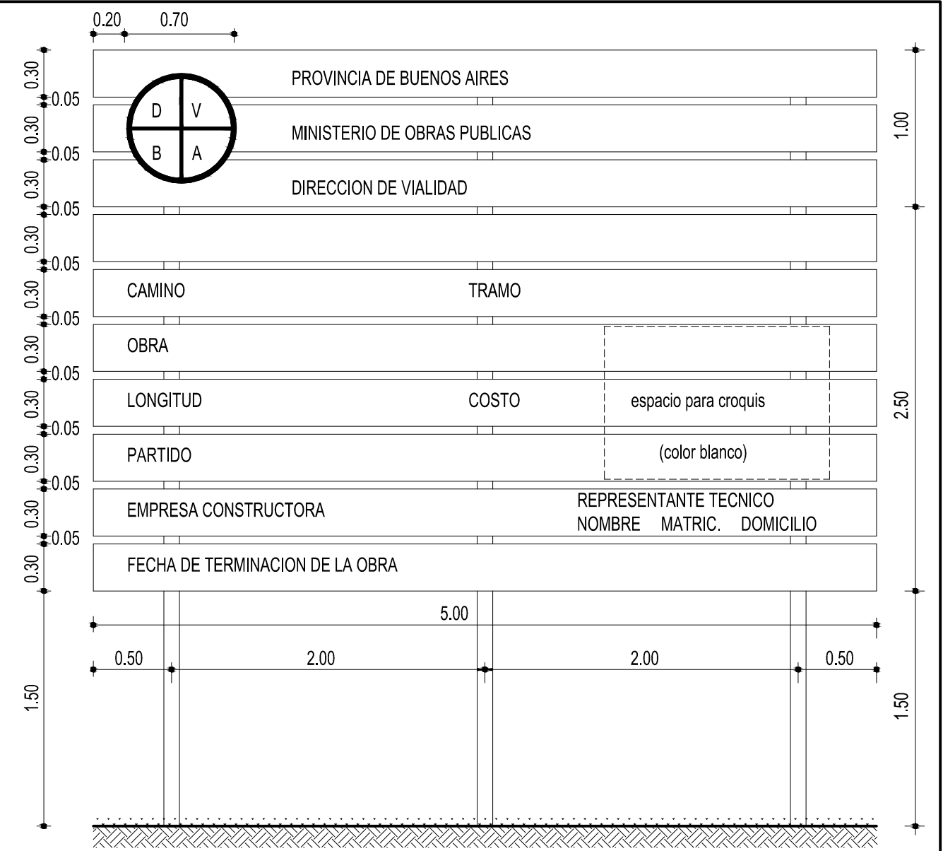
VISTA ESC. 1:30
