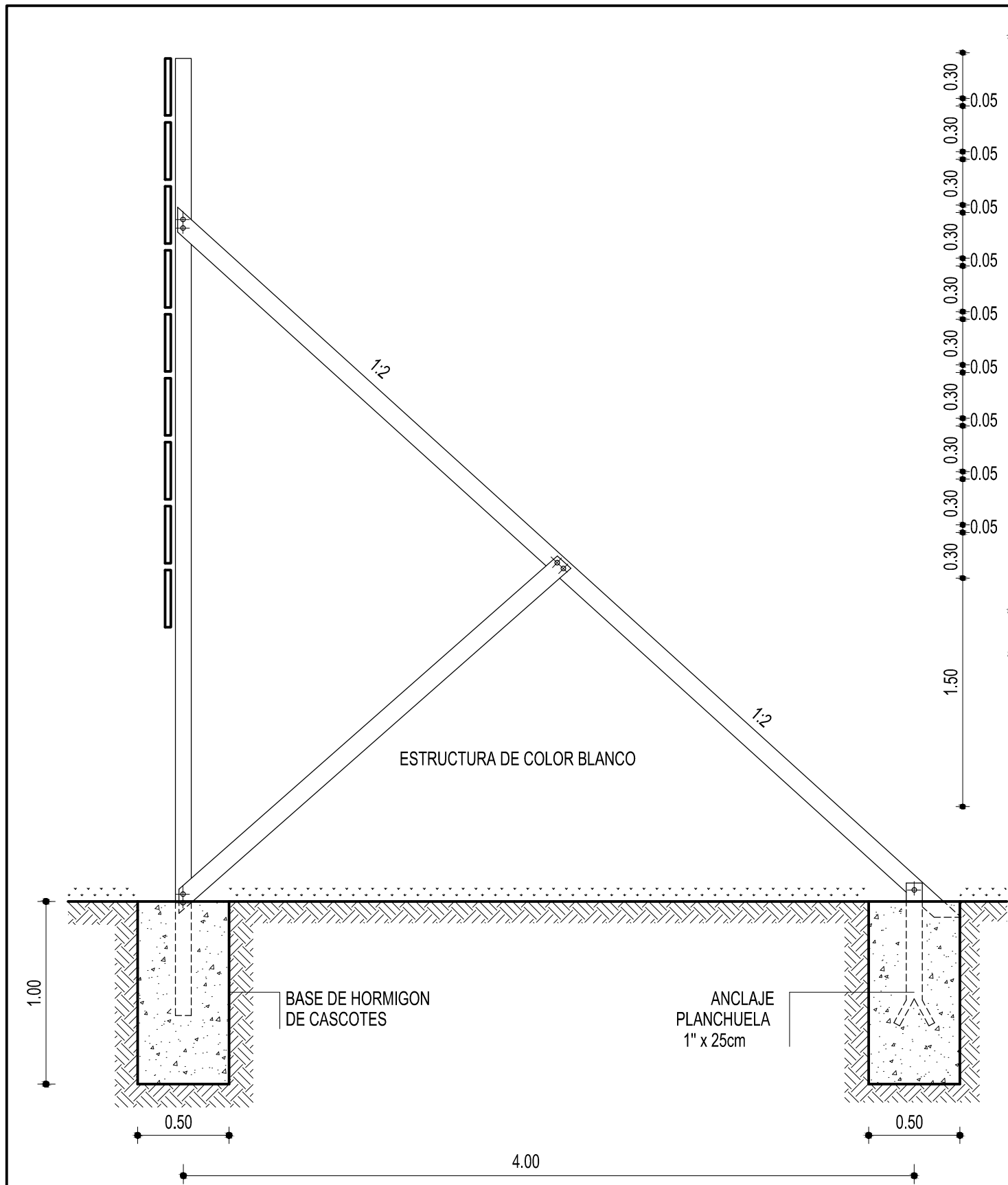
SECCION ESC. 1:25
